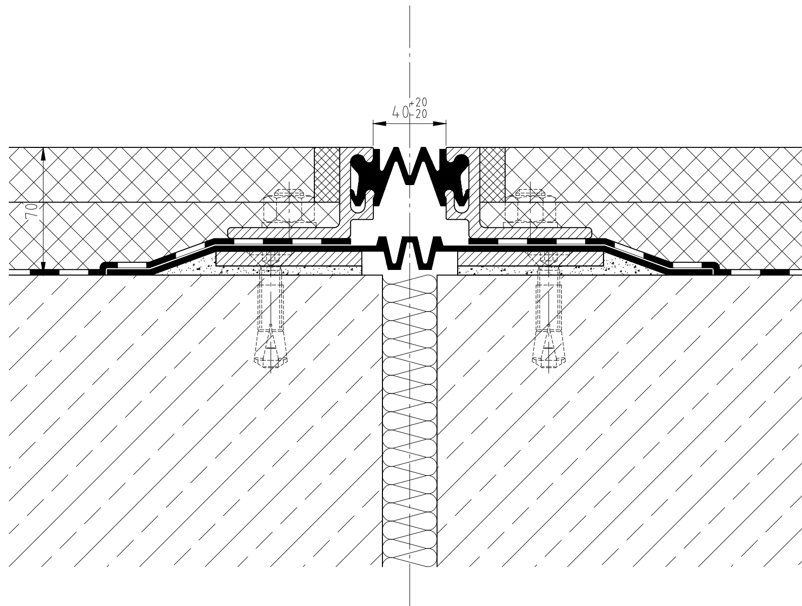
Dehnfugenonstruktion FK 50 - befahrbar ungedämmt
