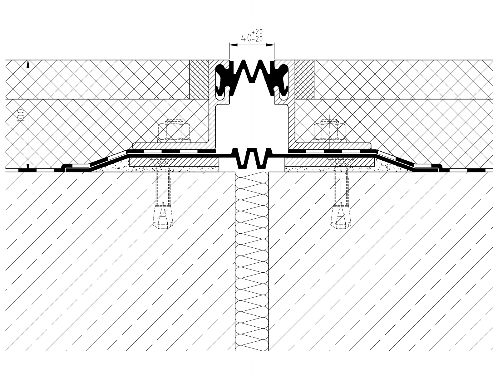
Dehnfugenonstruktion FK 80 - befahrbar ungedämmt
