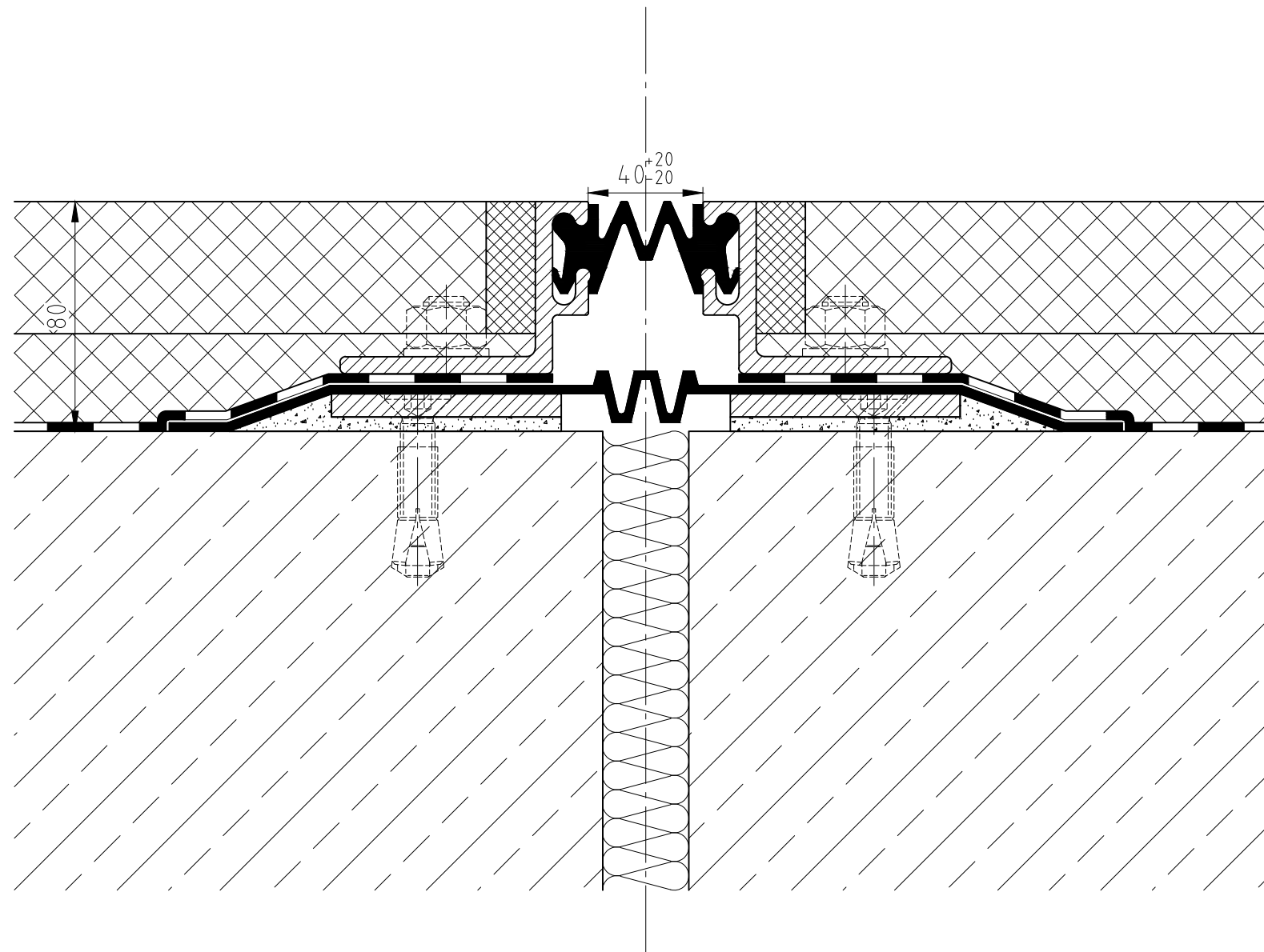
Dehnfugenonstruktion FK 60 - befahrbar ungedämmt
