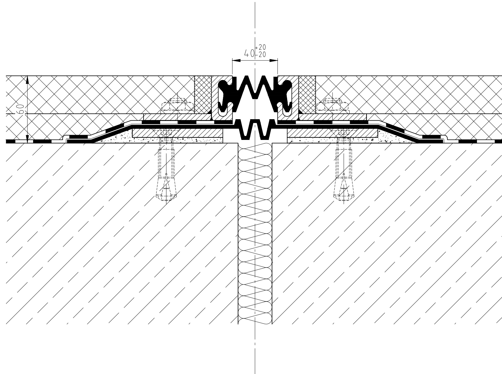
Dehnfugenkonstruktion FK 40 - befahrbar ungedämmt
